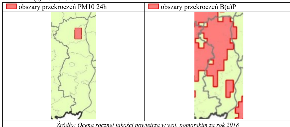
Rysunek 8 Obszary przekroczeń norm jakości powietrza na obszarze Powiatu Tczewskiego PM10 i B(a)P w 2018r.
